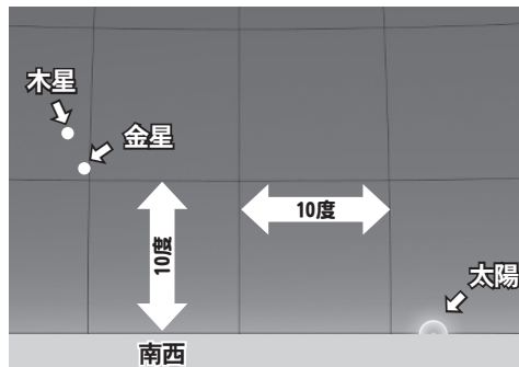
日没後の金星と木星の位置
