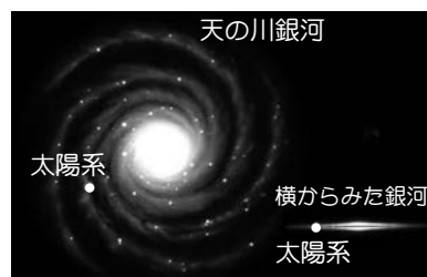
銀河系を上からと横からみた図
