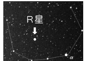
かんむり座R星
