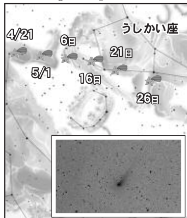
C/2015 V2 ジョンソン彗星(写真)と5月までの位置図
