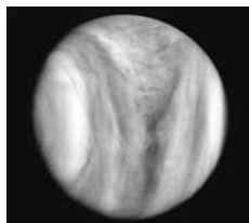
金星
