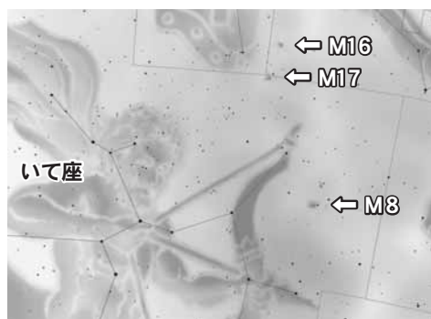
いて座付近の拡大図
