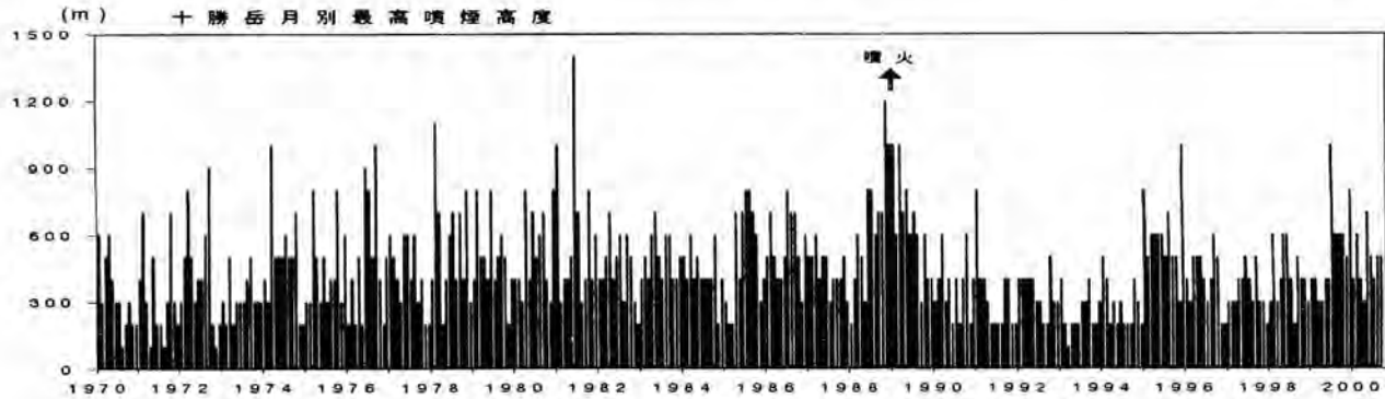
図2 月別最高噴煙高度
