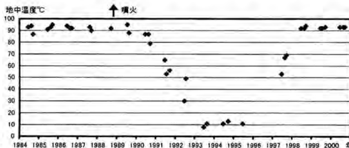
図5 振子沢噴気孔群の地中温度
