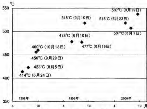
図3 62-2火口北西側内壁の噴気孔温度 注) 道立地質研究所のデータを含む
