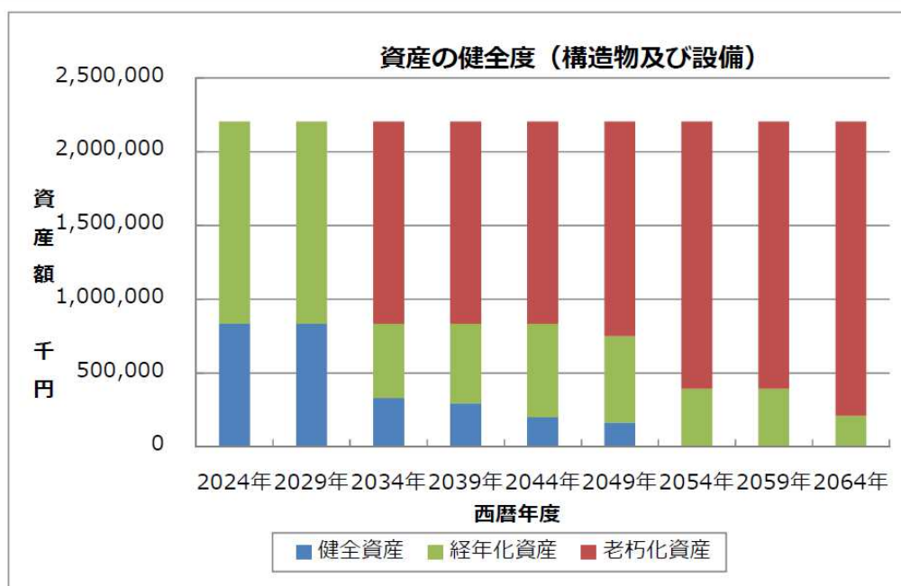
図 2.4 構造物及び設備の健全度
