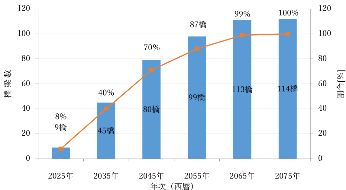
図1 上富良野町における建設後50年以上の橋梁数の推移
