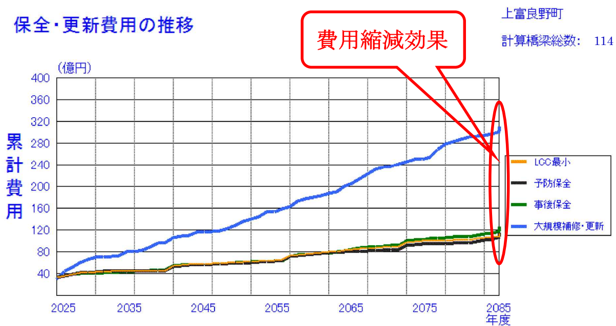
図4 保全・更新費用の推移（累計費用）
