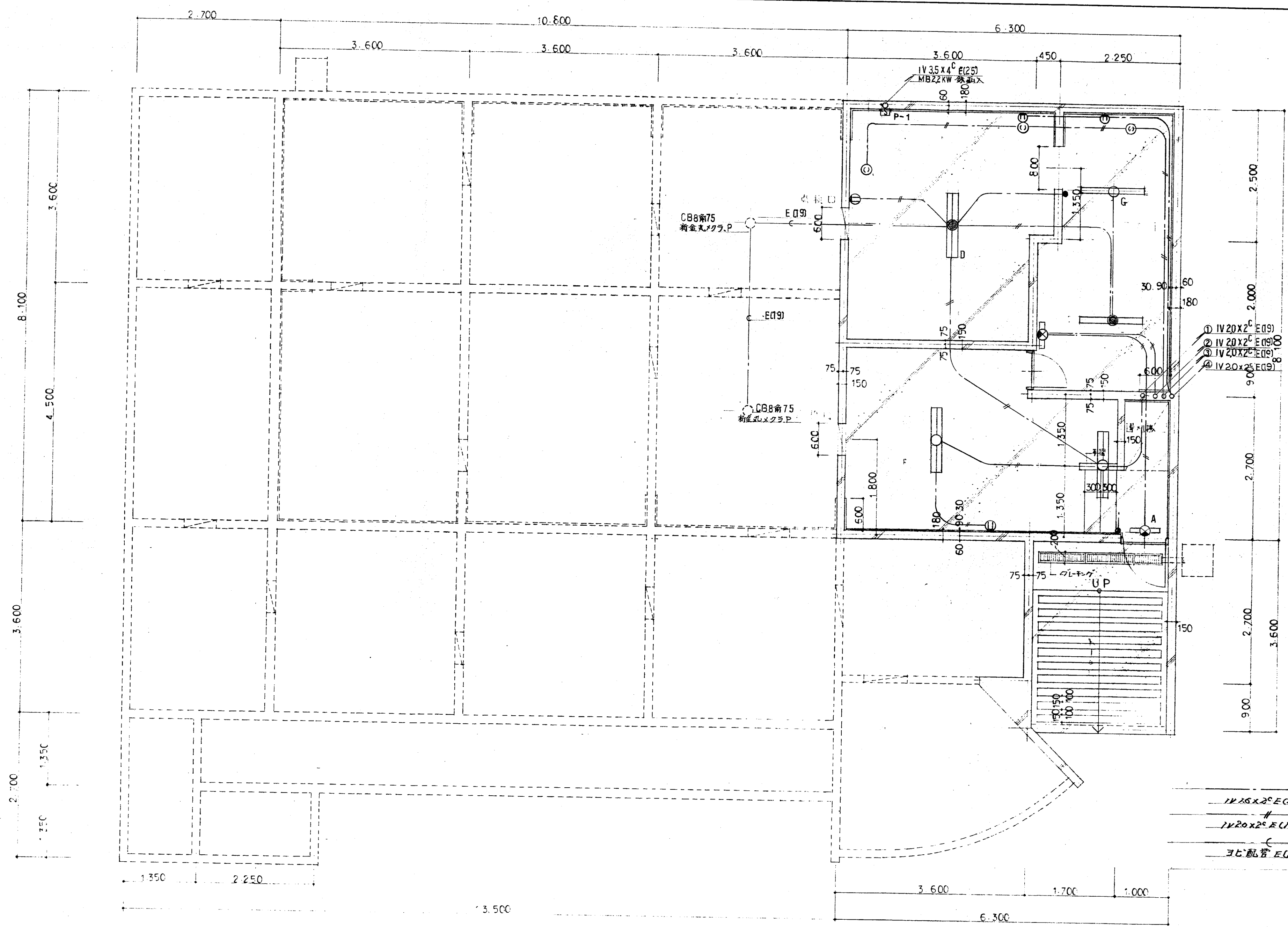
地階照明系統図 S=1/50
