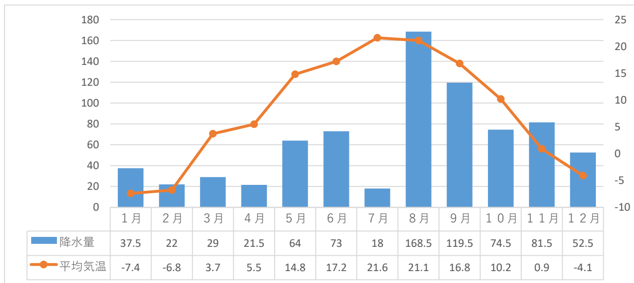
2019年の状況(旭川地方気象台ホームページより)
