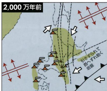
北海道の形成過程で隆起し エリア西側の山々が誕生した
