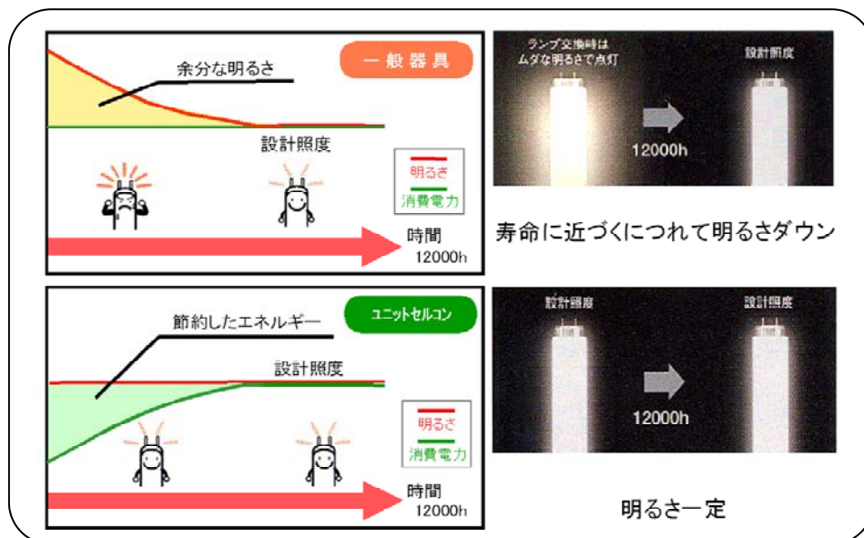
図 5-3-5 初期照度補正制御の概要
