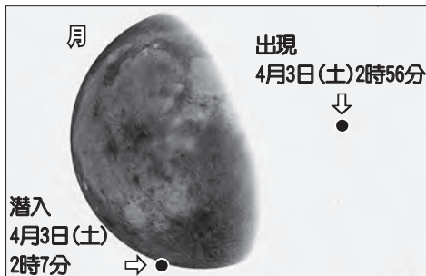
星食時のへびつかい座のθ星の位置
