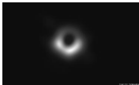
M87銀河の中心にあるブラックホール
