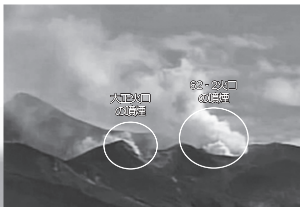
十勝岳 北西側から見た火口の状況
