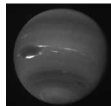
青々とした美しい姿の海王星
