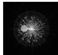
明るく輝く新星
