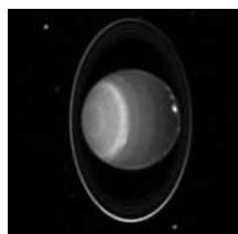
自転軸が傾いている天王星
