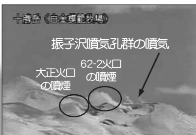
十勝岳 北西側から見た火口の状況
