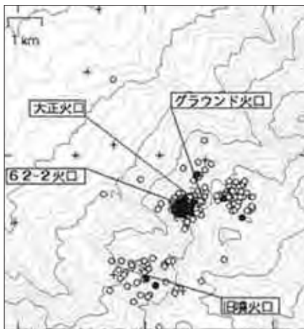
十勝岳の火山性地震の震源分布 ○印：2012年1月~12月の震源 ●印：2013年1月の震源
