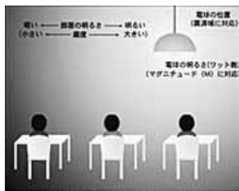
第1図 震度とマグニチュードの関係
