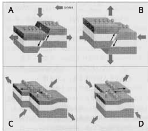
第1図 断層の種類
