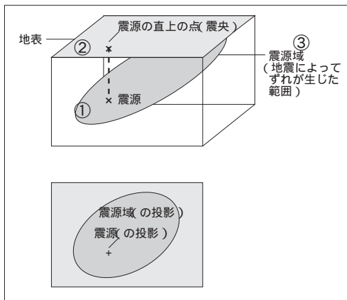
第2図 震源・震源域
