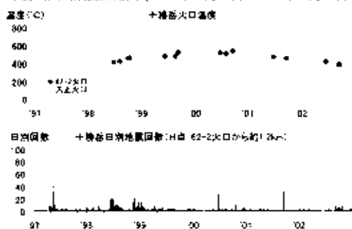
十勝岳火山活動経過図(1997年1月1日~2002年12月31日)
