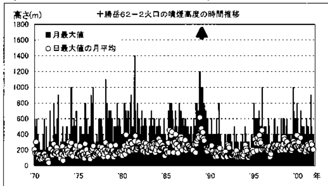
棒グラフ：月別最大噴煙高度(火口上の高度、単位m) 白丸：日別最大噴煙高度の月平均値(火口上の高度、単位m) 上矢印：1988~1989年の噴火活動
