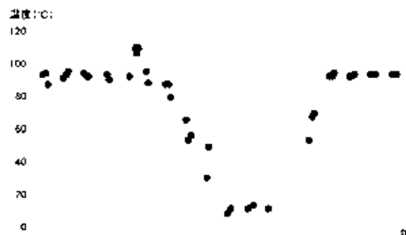
図3 振子沢噴気孔群における地中温度（50cm深）の推移 上矢印は1988～1989年の噴火活動を示す。
