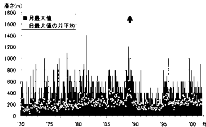
図1 62・2火口の噴煙高度の推移（1970年1月～2001年9月26日） 棒グラフ：月別最大噴煙高度（火口上の高度、単位m） 白丸：日別最大噴煙高度の月平均値（火口上の高度、単位m） 上矢印：1988～1989年の噴火活動
