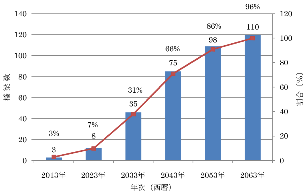
図-1 上富良野町における建設後 50 年以上の橋梁数の推移
