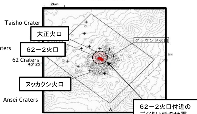
十勝岳 火山性地震の震源分布 (2012年12月~2019年11月5日10時)
