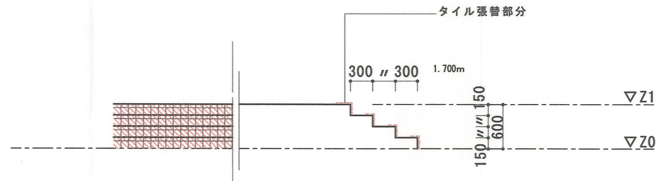
玄関ポーチ断面図
